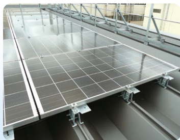
折版屋根設置事例
